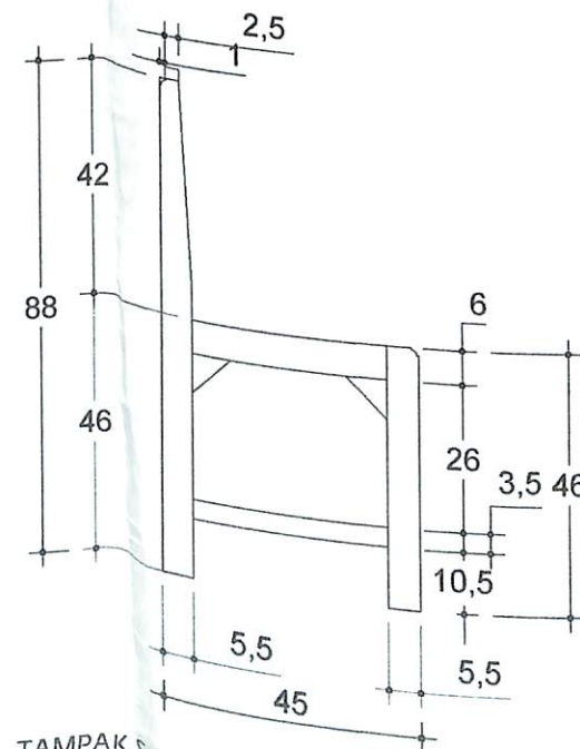
TAMPAK SAMPING KURSI GURU SEKALA: 1:15
