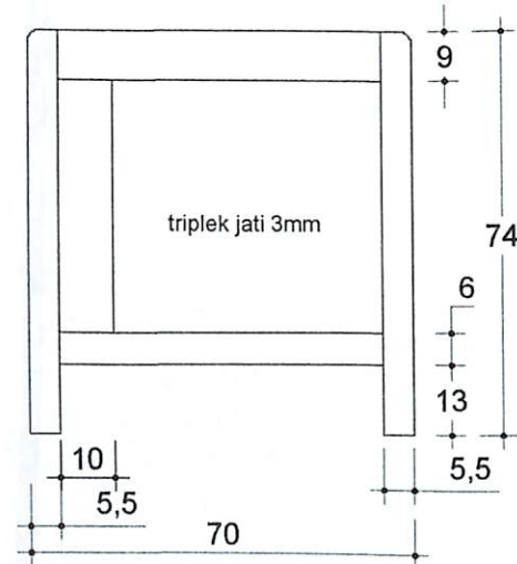
TAMPAK SAMPING MEJA GURU SEKALA: 1:15
