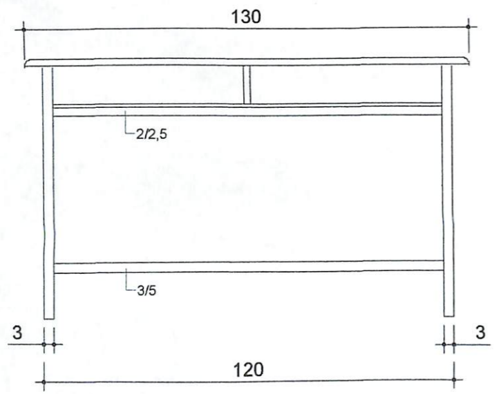
TAMPAK DEPAN MEJA MURID SEKALA: 1:15
