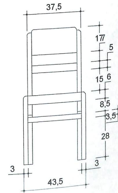
TAMPAK DEPAN KURSI GURU SEKALA: 1:15
