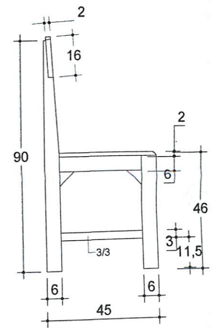
TAMPAK SAMPING KURSI MURID SEKALA: 1:15
