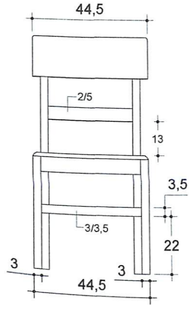
TAMPAK DEPAN KURSI MURID SEKALA: 1:15
