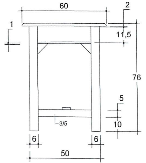
TAMPAK SAMPING MEJA MURID SEKALA: 1:15
