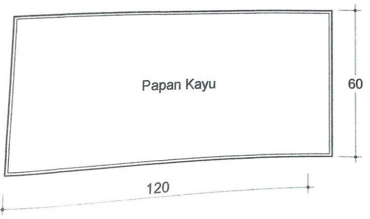
TAMPAK ATAS MEJA MURID SEKALA: 1:15
