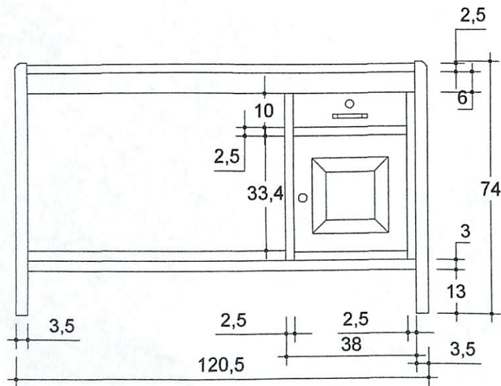
TAMPAK DEPAN MEJA GURU SEKALA: 1:15
